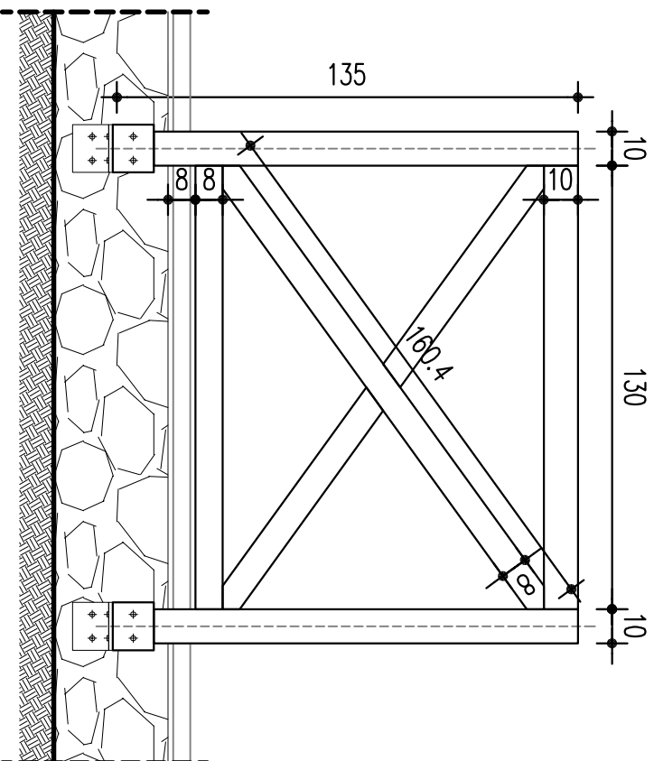
ΑΕΙΤΟΜΕΡΕΙΑ ΚΑ. 1:20
